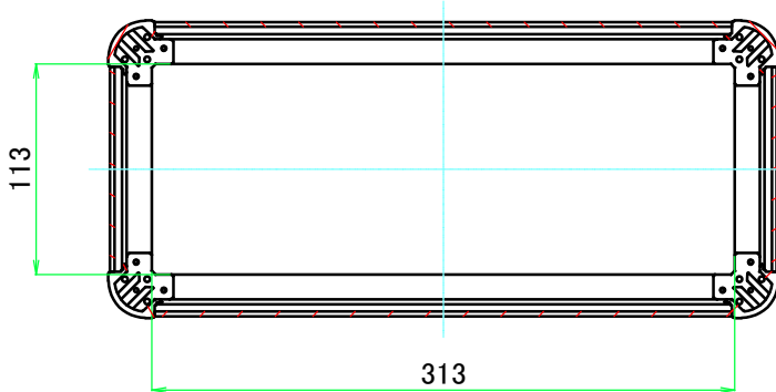
C-C ( 1 : 4.5 )
