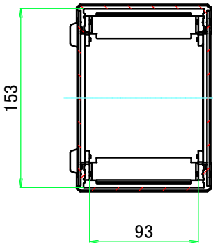
A-A ( 1 : 4.5 )
